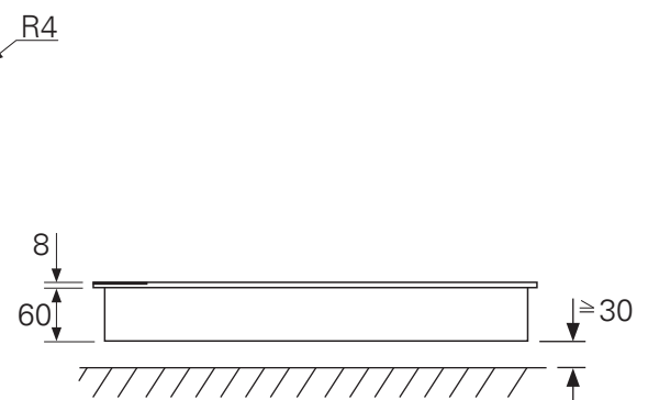
Gerätemaße TYE3000TL Frontansicht
