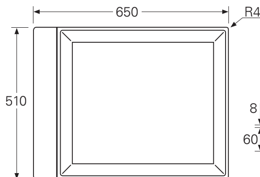
Gerätemaße TYE3000TL Draufsicht
