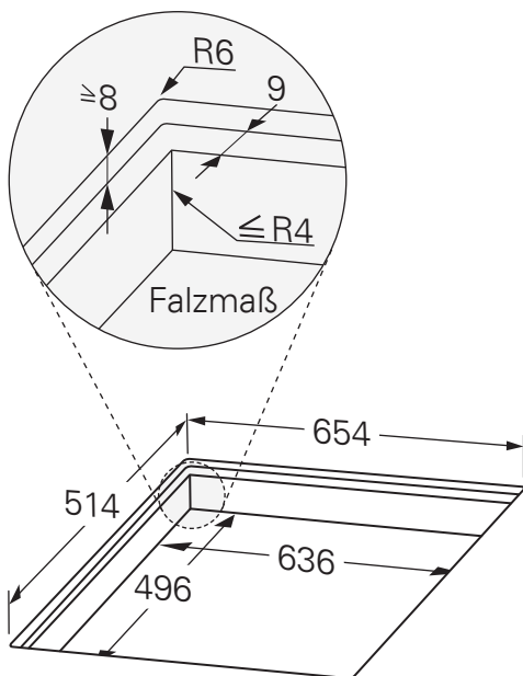
flächenbündiger Einbau (empfohlen)
