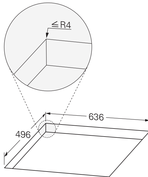
aufliegender Einbau
